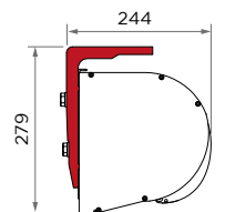
Rubis & Rubilux - Pose plafond -
