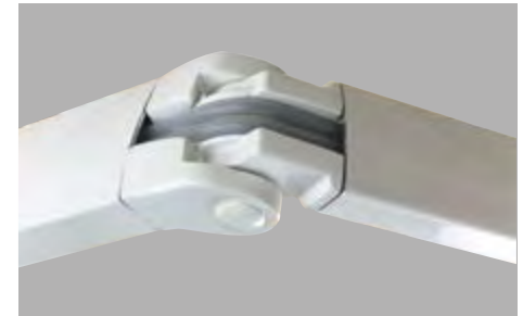
Bras en aluminium thermolaqué munie d'un double câble gainé. Les bras sont testé à 20 000 cycles.
