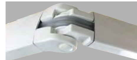
Bras en aluminium thermolaqué munie d'un double câble gainé. Les bras sont testé à 20 000 cycles.
