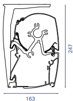
B24 ELITE / PRESTIGE montage au plafond
