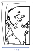
B27 montage au plafond
