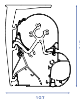
B25 ELITE / PRESTIGE VOLANT montage au plafond
