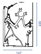
B27 ELITE / PRESTIGE montage murale
