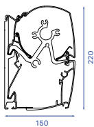
B24 ELITE / PRESTIGE montage murale
