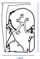
B25 ELITE / PRESTIGE montage au plafond
