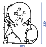
B25 ELITE / PRESTIGE VOLANT montage murale
