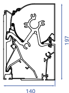
B27 montage murale
